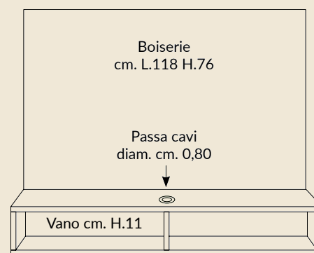
Art. 371347 Boiserie con porta tv e video cm. L.118 P.35 H.91 € 1.014,00
