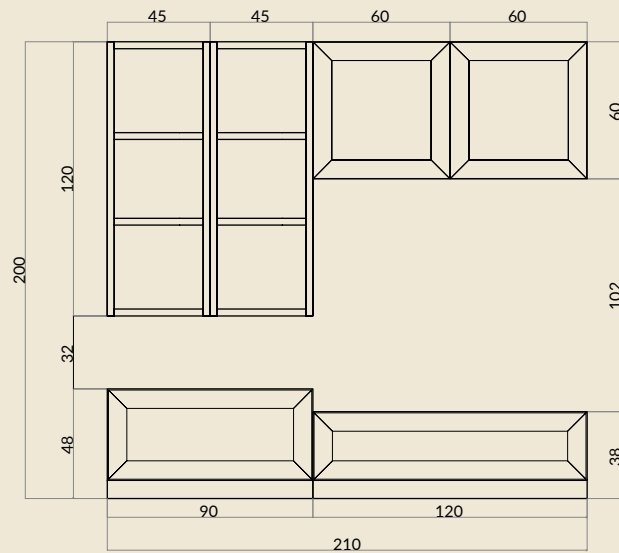
Art. 121056 COMPOSIZIONE. cm. L. 210 P. 57/38 H. 200 € 3.353,00
